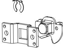
Staffa con perno quadrato 16 mm + omega Bracket with square pin 16 mm + omega
