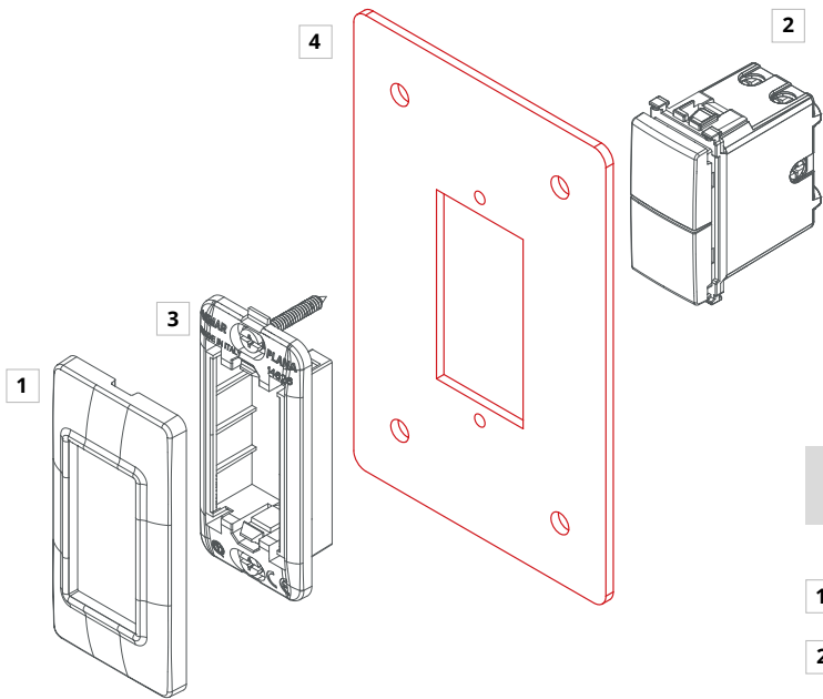
Kit placca con interruttore Vimar per argano Plate kit with Vimar switch for winch
