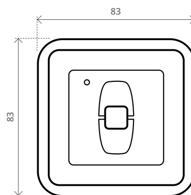
Telecomando monocanale da parete per il controllo di 1 tapparella o tenda da sole o di un gruppo Single channel wall remote control for controlling rolling shutter or awning or one group
