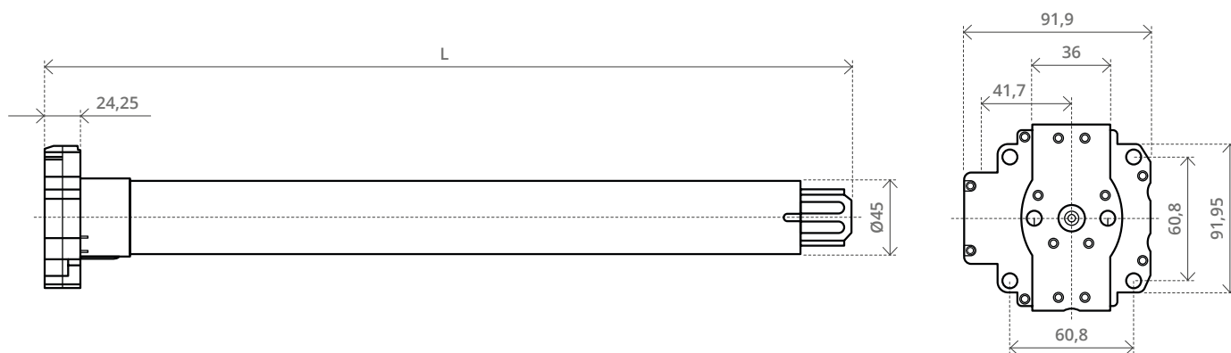
Motori finecorsa meccanico con manovre di soccorso Ø50mm Mechanical limit switch motor with manual override Ø50mm
